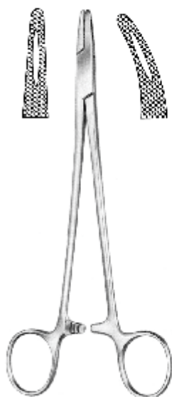
MAYO-HEGAR
