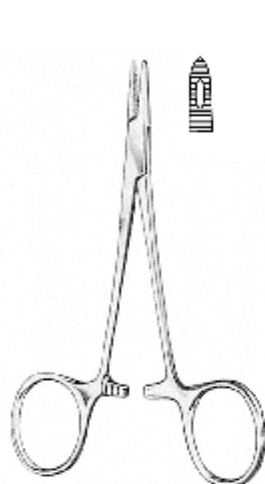
DERF 22.0010.12 12.0cm
